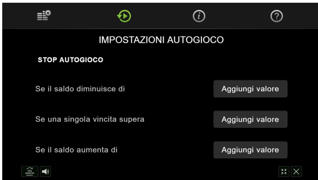
Fig. 3 Impostazioni Autogioco
