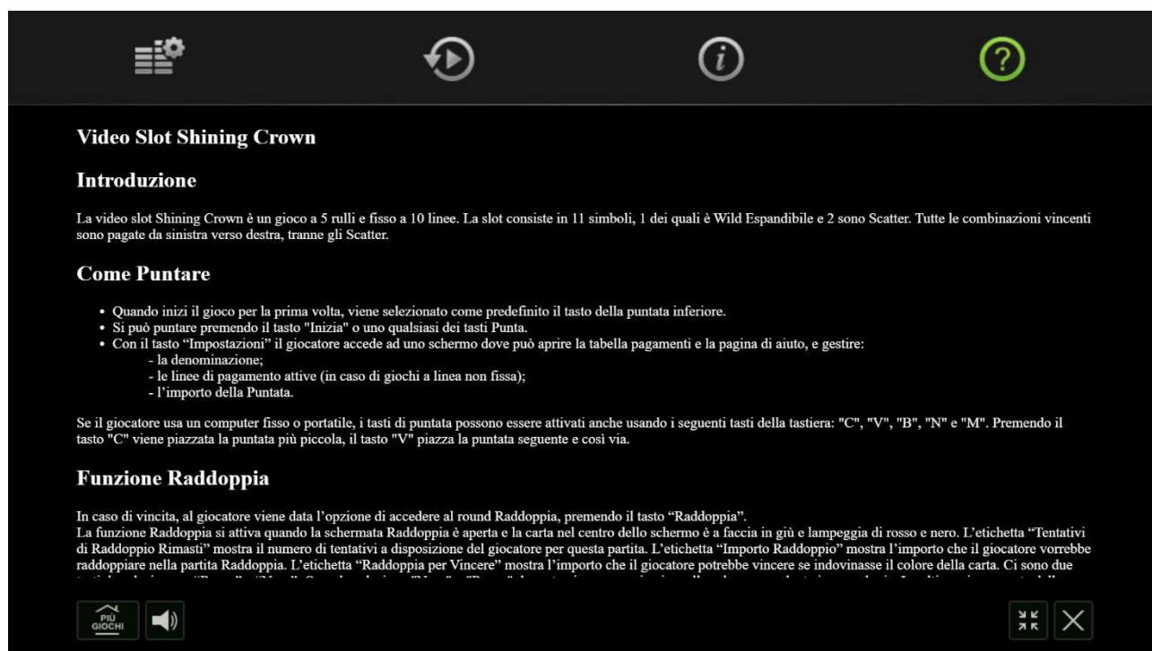
Fig. 5 Aiuto
